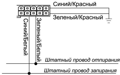
Схема 1. 3-проводная система с отрицательной полярностью (большинство японских автомобилей)
