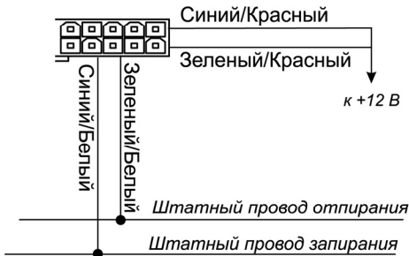
Схема 2. 3-проводная система с положительной полярностью (большинство автомобилей GM)
