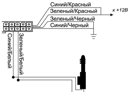
Схема 6. Установка дополнительных электроприводов
