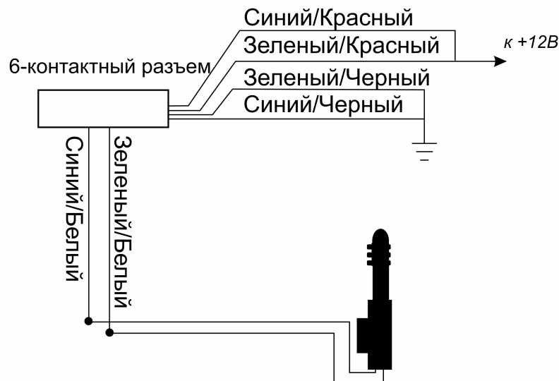
Схема 6. Установка дополнительных электроприводов
